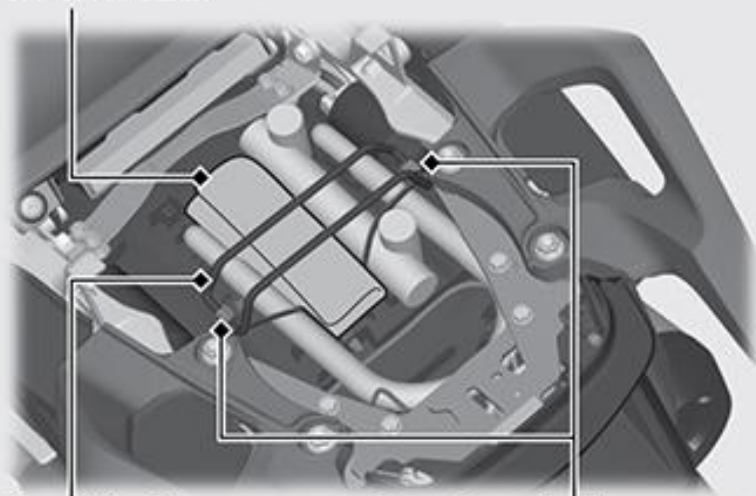
Cinghia in gomma A Punti di aggancio
